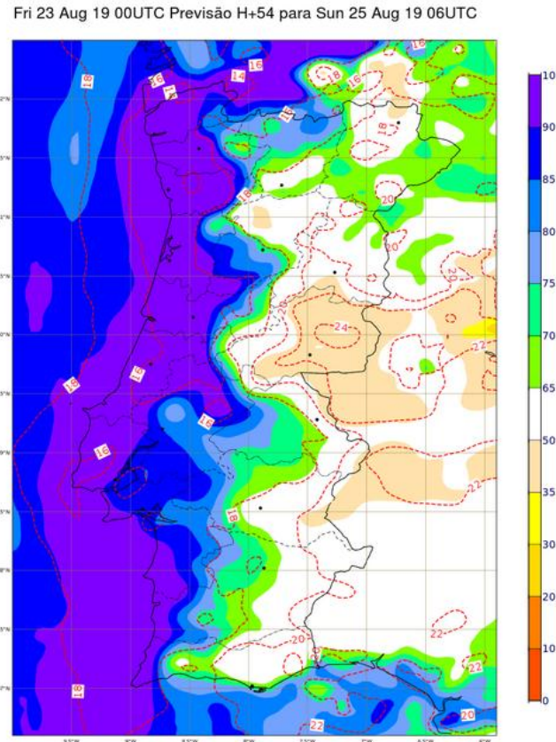
HR 06UTC noite 24/25 Humidade Relativa (%) a 2m Fri 23 Aug 19 00UTC Previsão H+54 para Sun 25 Aug 19 06UTC
