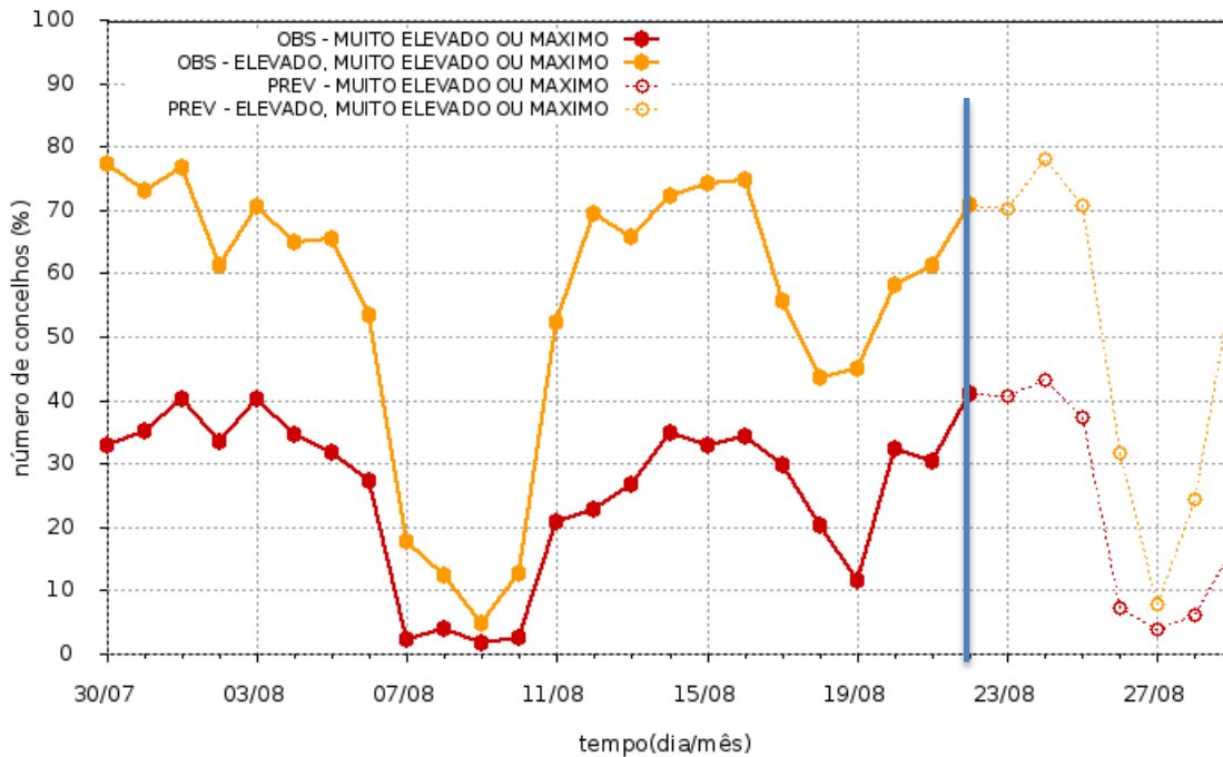
Número de Concelhos (%) em Risco Elevado, Muito Elevado ou Máximo Observação: 30jul a 22ago - Previsão: 23ago a 29ago
