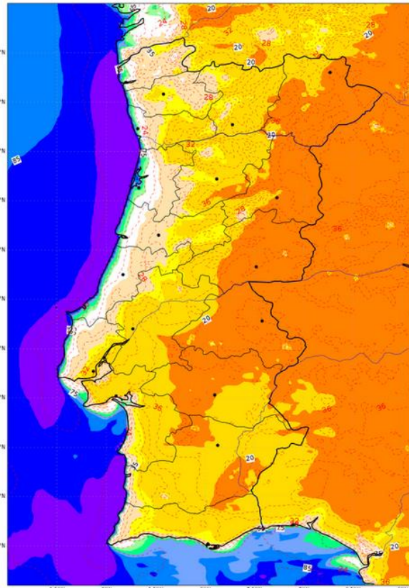
AROME HR 15UTC Humidade Relativa (%) a 2m Fri 23 Aug 2019 00 UTC Previsão H+39 para Sat 24 Aug 2019 15 UTC
