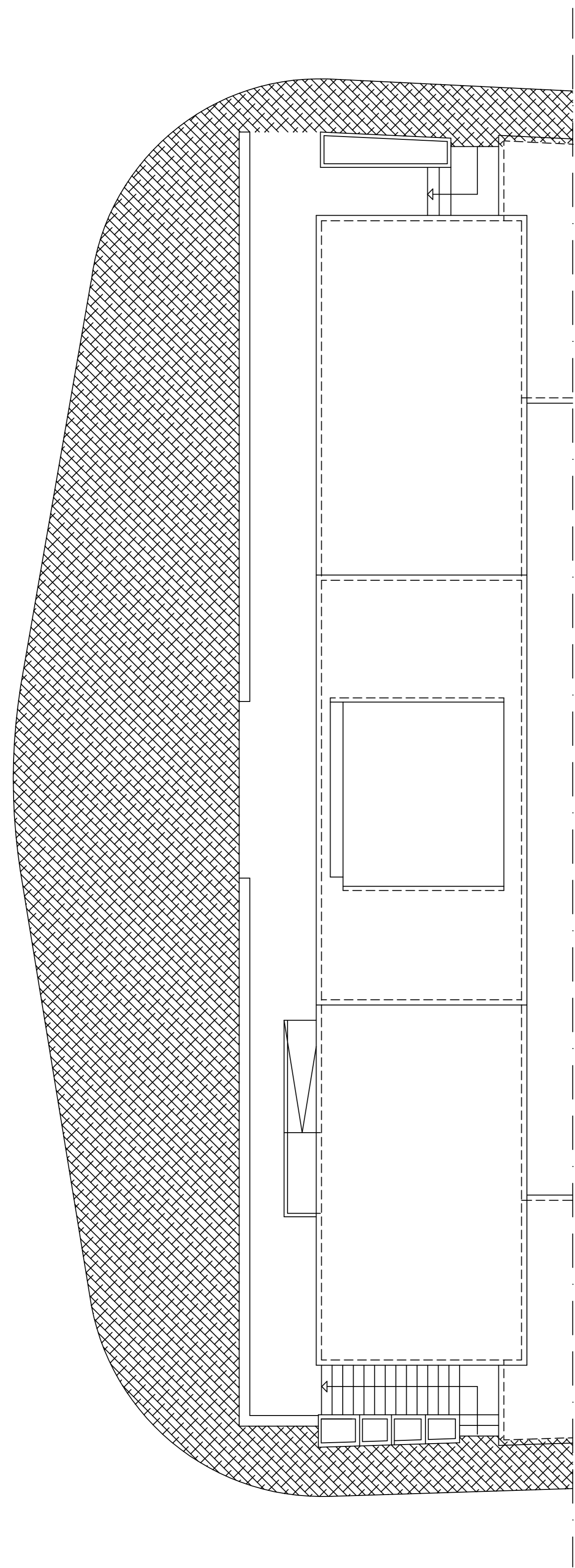
Planta parcial das coberturas
